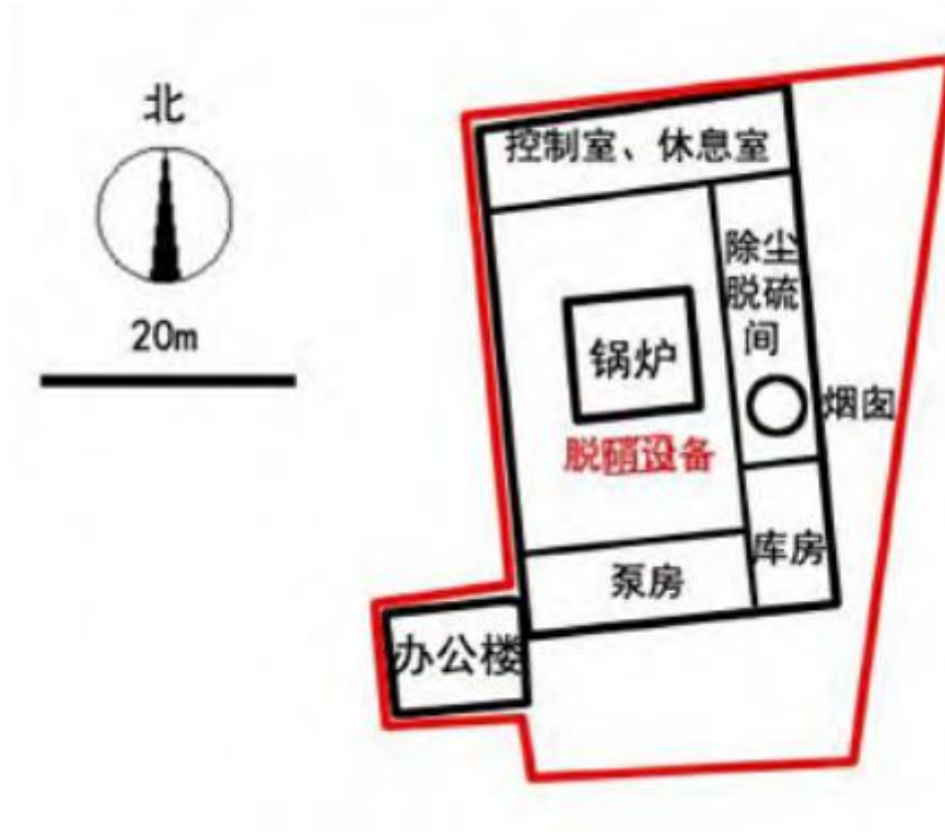
图 2.3 本次改造后锅炉房厂房内平面布局图
