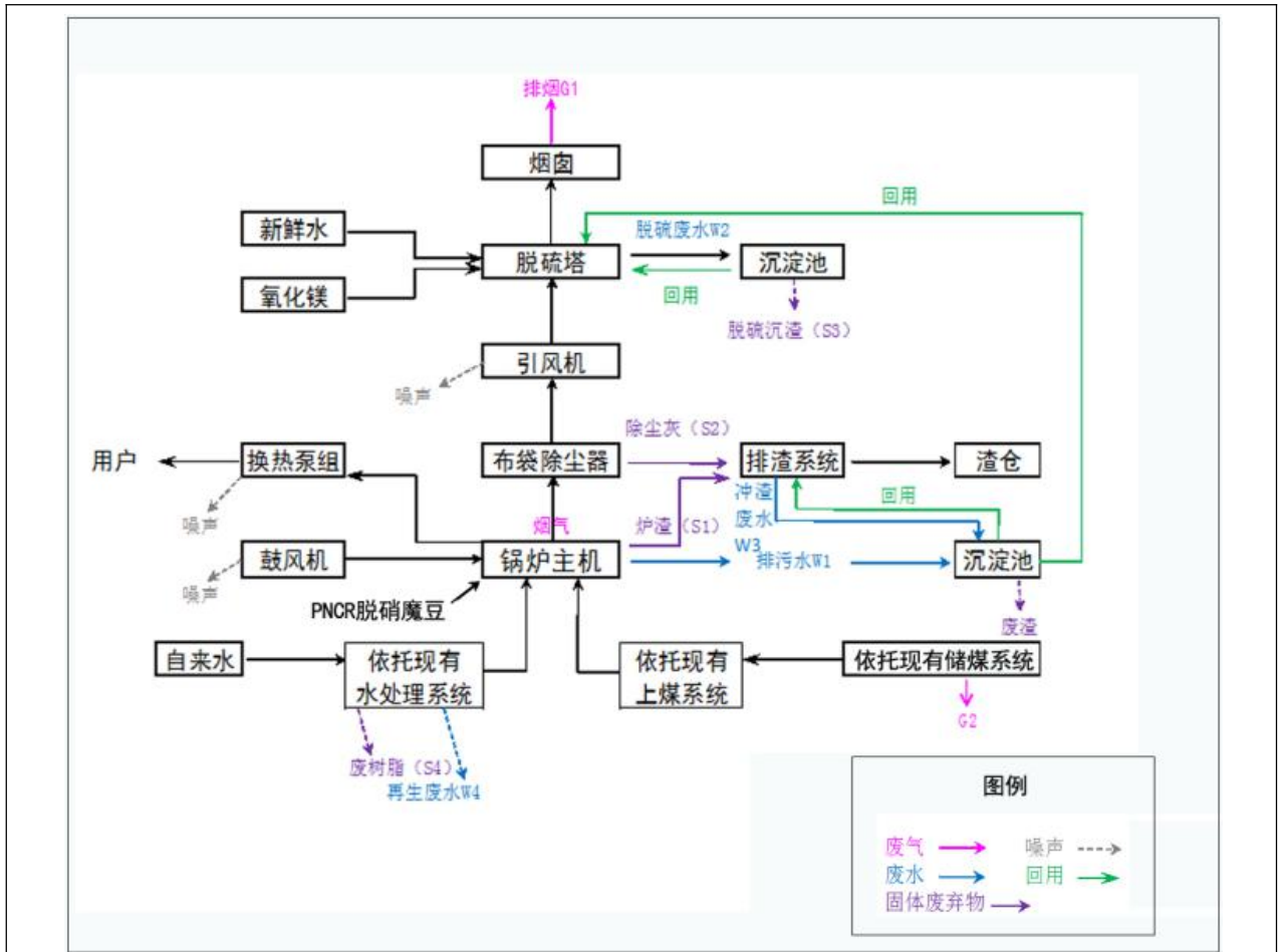
图 2.4 工艺流程图
